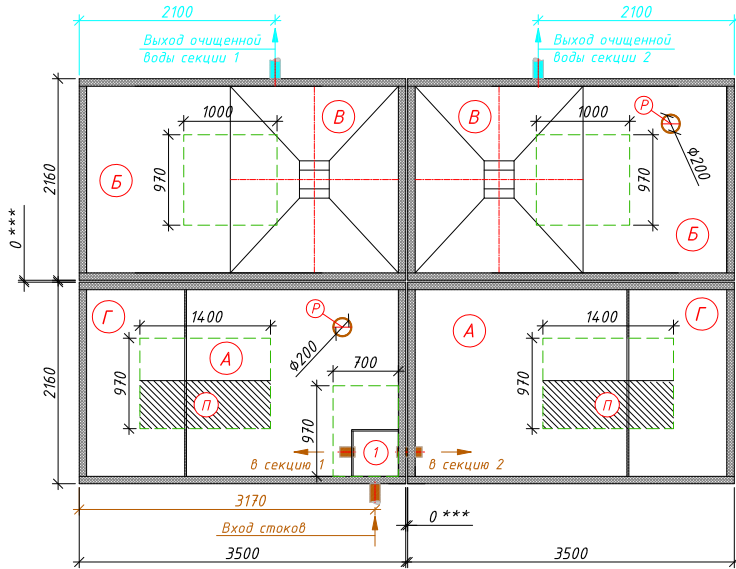
Схема станции
